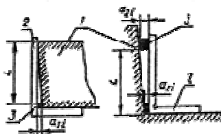
1 - проверяемое изделие; 2 - угольник; 3 - щуп, концевая мера, линейка
