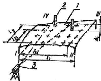
1 - проверяемая поверхность; 2 - линейка; 3 - нивелир
