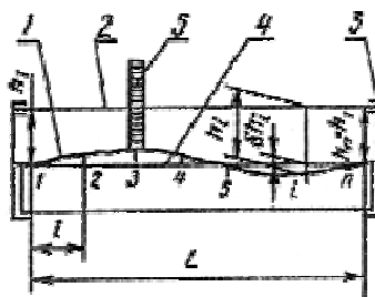
1 - проверяемая поверхность; 2 - струна; 3 - опоры для натяжения струны; 4 - условная прямая; 5 - линейка для снятия отсчета
