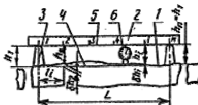
1 - проверяемая поверхность; 2 - поверочная линейка, рейка; 3 - опорная призма; 4 - условная прямая; 5 - линия отсчета; 6 - индикатор
