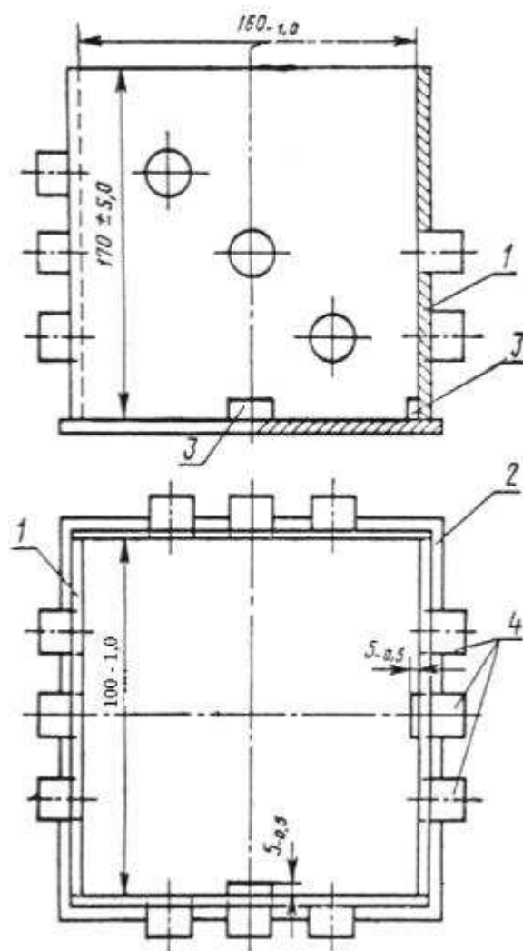
1 - стенка ванны; 2 - основание ванны; 3 - фиксатор; 4 - пьезоэлектрические преобразователи
