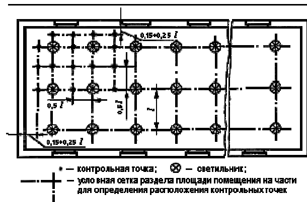
Рисунок А1 - Расположение контрольных точек при измерении минимальной освещенности помещения от светильников, принимаемых за точечные излучатели
