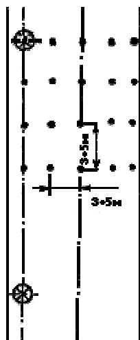
Рисунок А3 - Расположение контрольных точек при измерении средней освещенности в помещении
