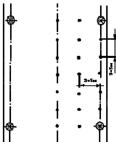
Рисунок А3 - Расположение контрольных точек при измерении средней освещенности в помещении
