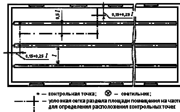
Рисунок А2 - Расположение контрольных точек при измерении минимальной освещенности помещения от светильников, принимаемых за линейные излучатели
