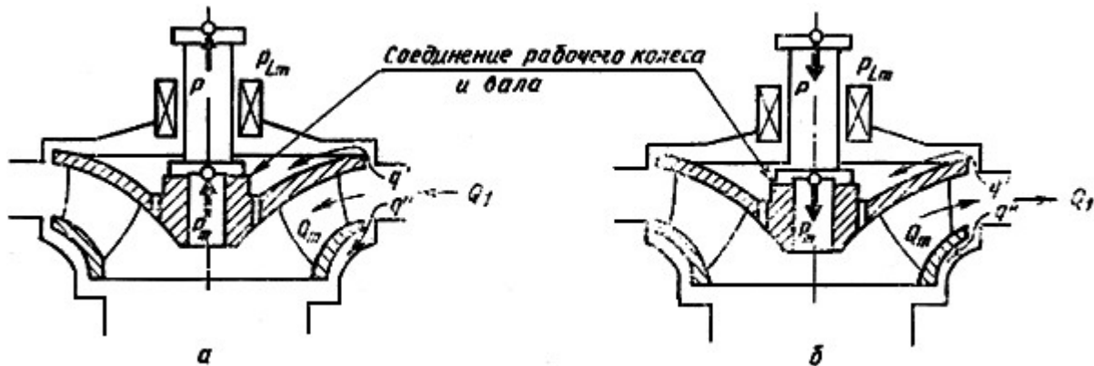
а - турбина; б - насос
