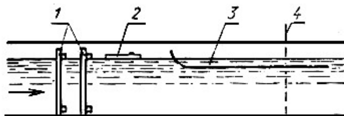
1 - решетки; 2 - плоты; 3 - подтопленный плот; 4 - измерительное сечение
