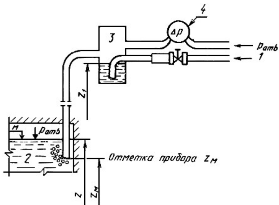
1 - сжатый воздух; 2 - конец трубки; 3 - контрольный сосуд; 4 - измеритель перепада давлений
