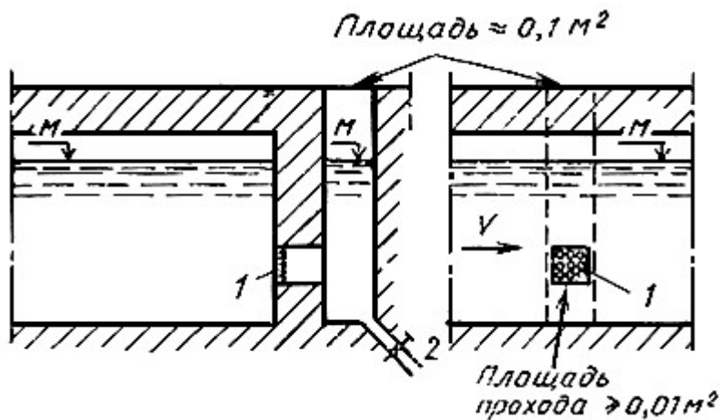
Измерительный колодец
