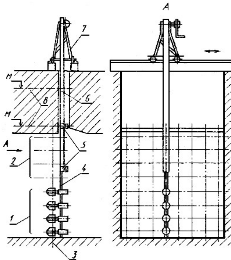
1 - положение 1; 2 - положение 2; 3 - измерительное сечение; 4 - штанга крепления расходомеров; 5 - направляющие зажимы; 6 - профильная штанга; 7 - тележка; 8 - уровень воды предельный
