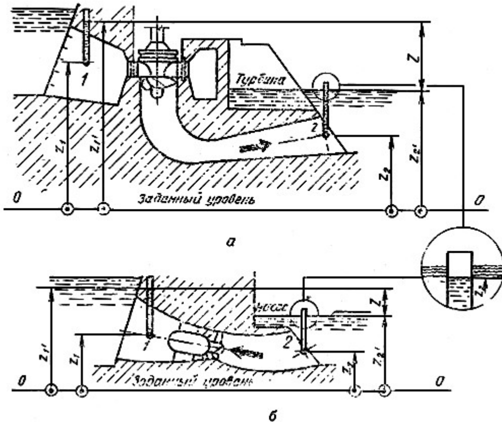
а - пропеллерная или поворотно-лопастная турбина; б - осевой насос
