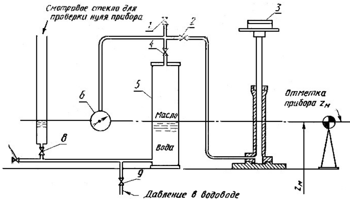
Градуировка пружинного манометра или преобразователя давления в процессе испытания
