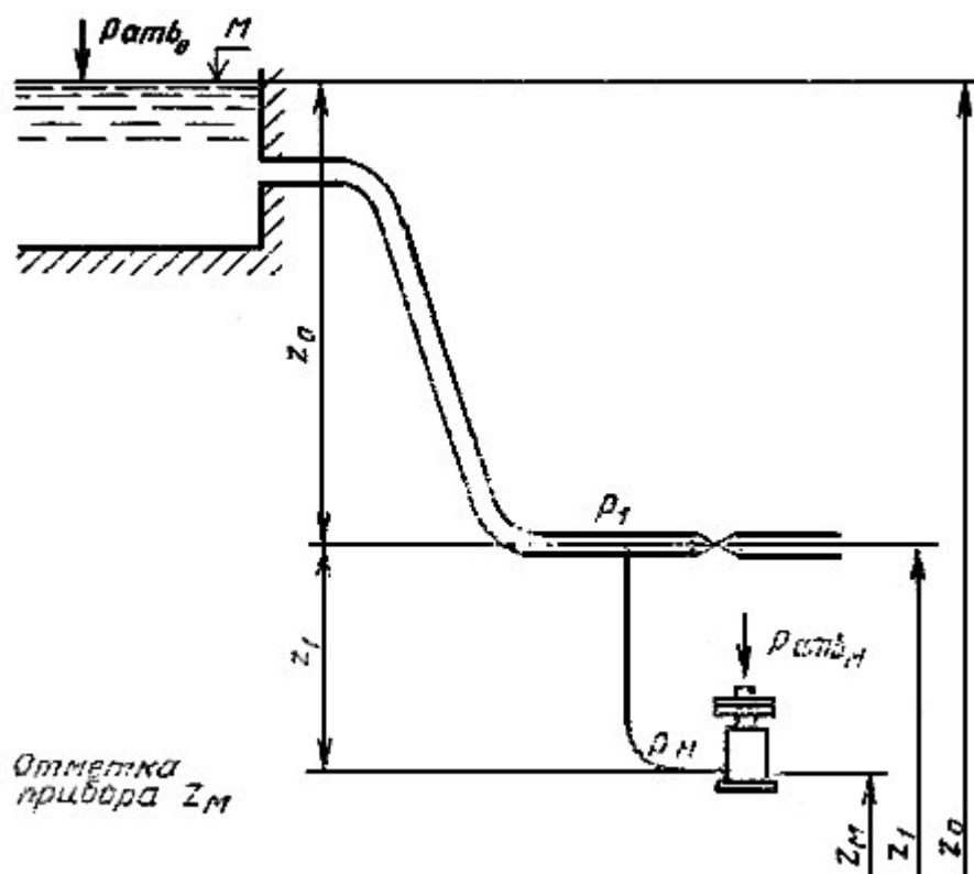
Схема проверки манометра
