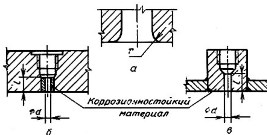
Примеры отверстий для отбора давления
