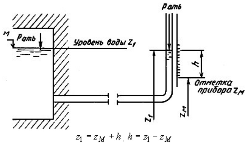
Схема измерения уровня водомерной трубкой
