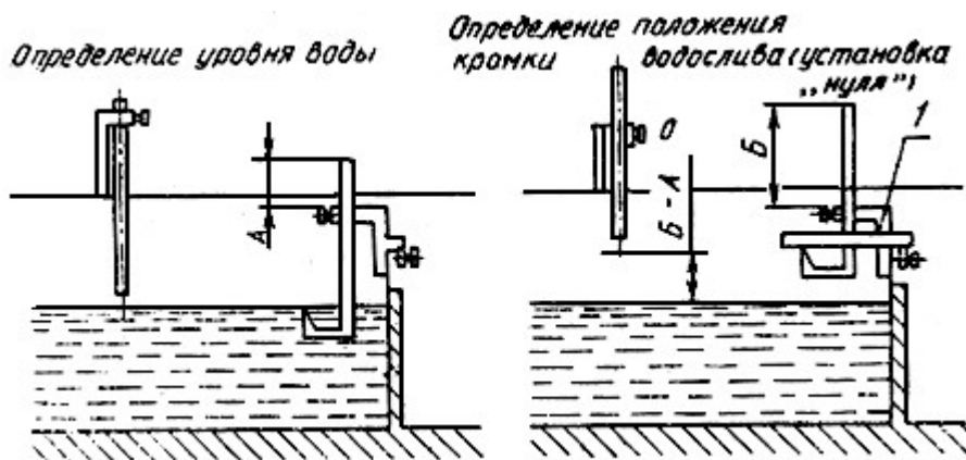
Узел прибора при определении положения кромки водослива "установки уровня гребня водослива"
