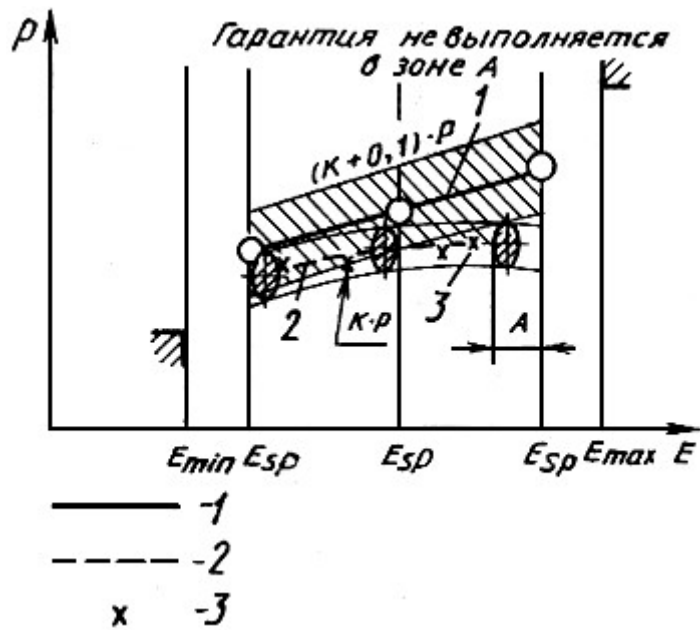
1 - кривая по требованиям технического задания; 2 - кривая по результатам измерений; 3- результат измерений
