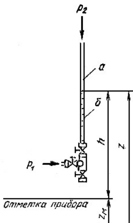
3. Манометр с U-образной трубкой
