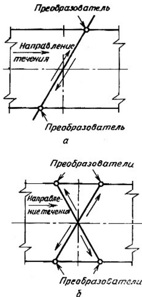
а - однолучевая система с последовательной передачей сигналов; б - двухплоскостная однолучевая система с синхронной или последовательной передачей сигналов
