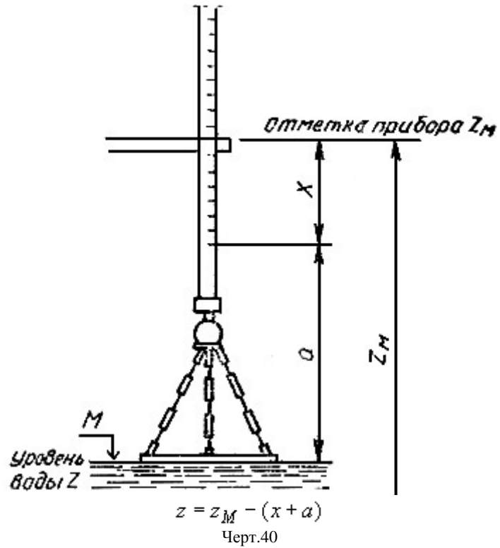
Пластинчатый уровнемер
