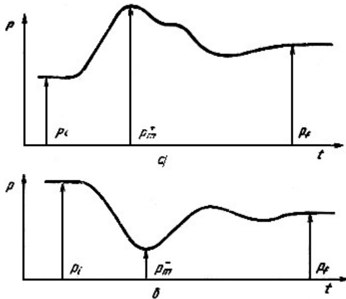
а - после внезапного сброса заданной нагрузки; б - после внезапного приложения заданной нагрузки
