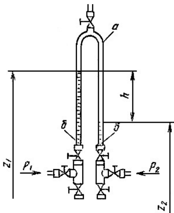
4. Манометр с перевернутой U-образной трубкой
