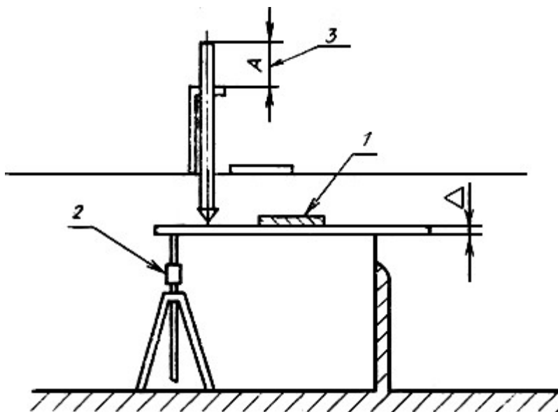
Определение положения кромки водослива (установка "нуля" в осушенном канале)
