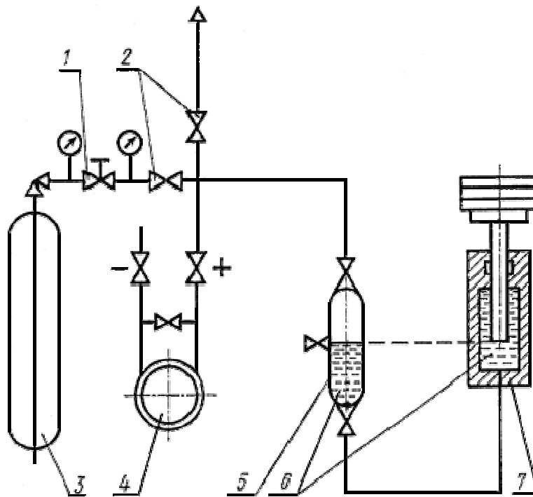
1 - редуктор; 2 - запорный вентиль; 3 - баллон со сжатым азотом; 4 - поверяемый преобразователь; 5 - разделительный сосуд; 6 - рабочая жидкость; 7 - грузопоршневый манометр
