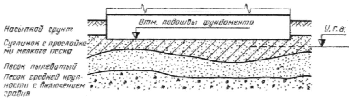
План расположения марок и эпюры перемещений
