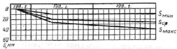
График развития перемещений
