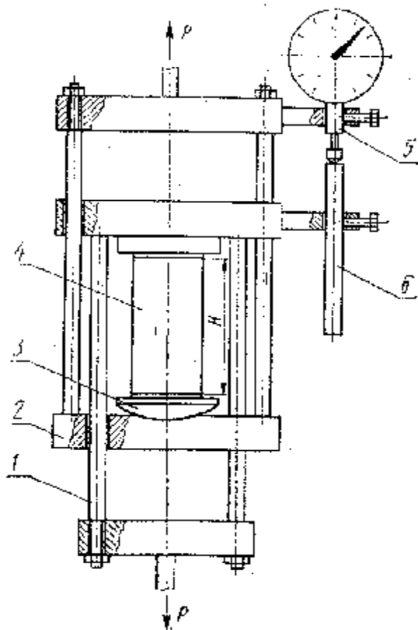
1 - нижняя траверса реверсора; 2 - верхняя траверса реверсора; 3 - шарнирная опора; 4 - образец; 5 - индикатор часового типа; 6 - упорный шток
