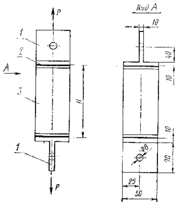
1 - Т-образная пластина; 2 - клей; 3 - образец
