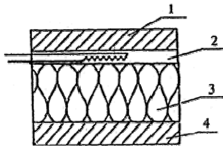
Рисунок А.1 - Схема прибора с одним тепломером
