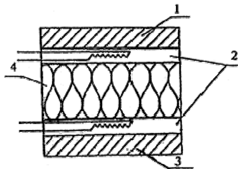
Рисунок А.2 - Схема прибора с двумя тепломерами
