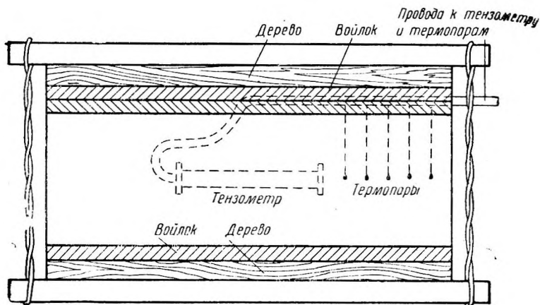
Фиг. 2. Схема устройства теплоизоляции образца и расположение приборов.
