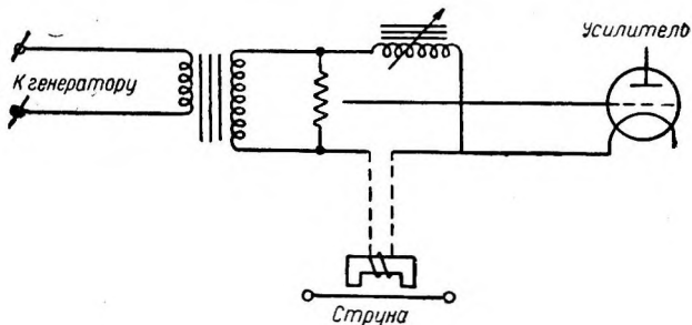
Фиг. 11: Схема моста Уитстона в установке 1930 г.
