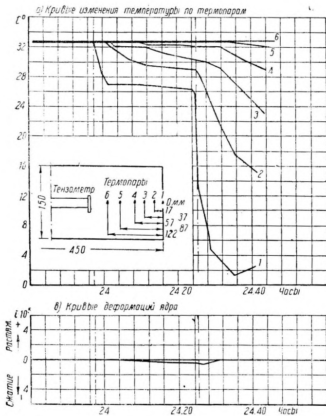
Фиг. 14. Влияние резного образования трещины на деформации ядра.
