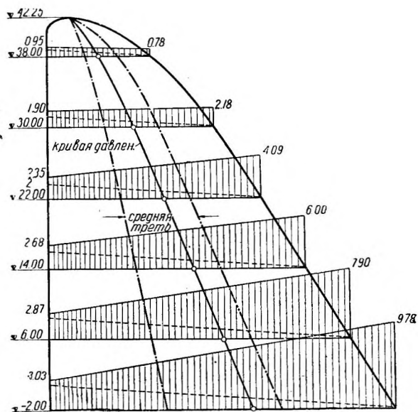
Фиг. 3. Кривая давления и эпюры нормальных напряжений для второй схемы загрузки (собственный вес и давление воды при отметке 51,20). Напряжения в \text{кг}/\text{см}^2 .
