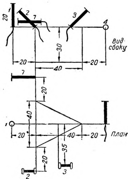
Фиг. 32. Схема расположения тонзометров на каркасе.
