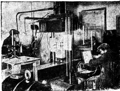
Фиг. 15. Параллельные наблюдения за деформациями бетонной призмы по струнному теле тензометру и зеркальным приборам Мертенса.
