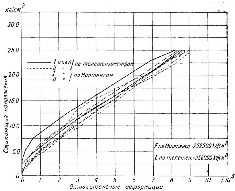
Фиг. 10. Кривые деформаций по приборам Мартенса и по телеметру, заложенному по оси призмы.
