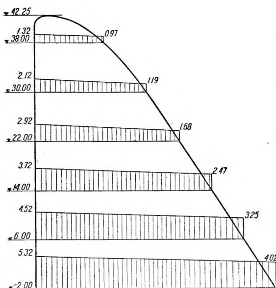
Фиг. 6. Эпюры нормальных напряжений \sigma_x для второй схемы загрузки (собственный вес и давление воды при отметке 51, 20). Напряжения в кг/см^2 .
