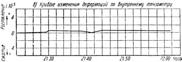
Фиг. 11. Влияние трещины на показания внутреннего тензометра. Направления трещины и прибора составляют угол около 60°.
