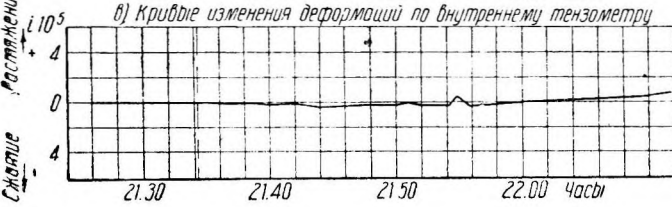
Фиг. 9. Влияние глубокой трещины на показания внутреннего тензометра. Трещина по направлению оси прибора.
