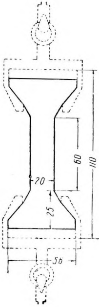
Фиг. 5. Бетонный образец для испытания на растяжение.
