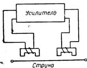
Фиг. 2. Схема двухмагнитного самовозбуждения.
