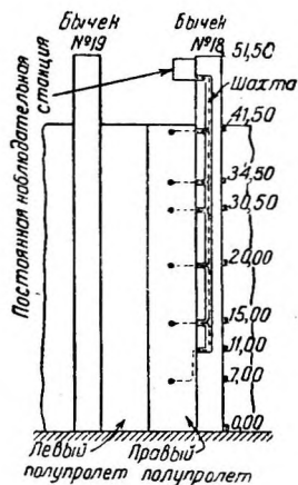
Фиг. 3. Схема прокладки кабелей от приборов, заложенных в плотину, к постоянной измерительной станции на бычке № 18.
