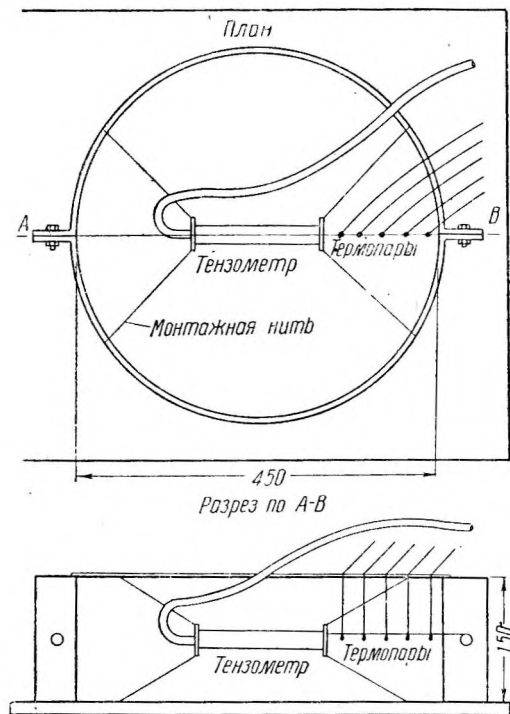
Фиг. 17. Схема монтажа приборов в форме перед бетонировкой.
