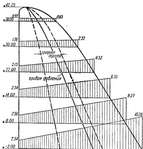
Фиг. 4. Кривая давления и эпюры нормальных напряжений \sigma_y для третьей схемы загрузки (собственный вес, давление воды при отметке 52,30 и давление наносов). Напряжения в \text{кг/см}^2 .
