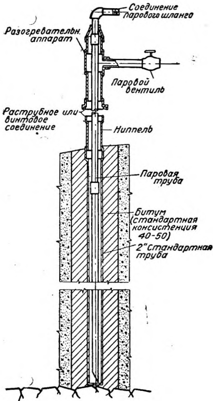
Фиг. 7. Аппарат для прогрева шпонок.
