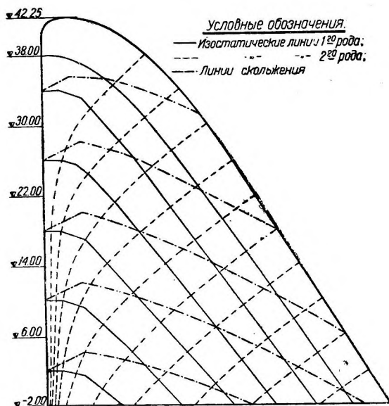
Фиг. 10. Изостатические линии и линии скольжения в теле плотины для второй схемы нагружения (собственный вес и давление воды при отметке горизонта 51, 20).
