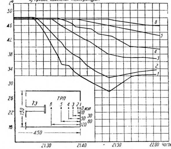
а) Кривые изменения температуры
