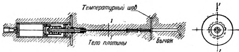
Фиг. 9. Струнный щелемер проф. Ю. А. Нилендера.
