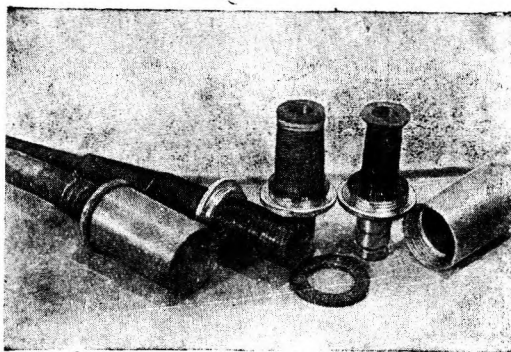
Фиг. 19. Термометры сопротивления.
