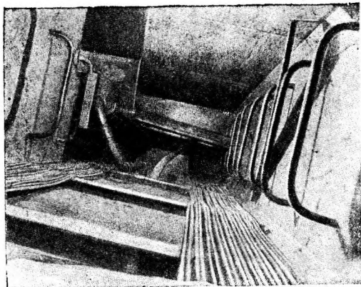
Фиг. 28. Шахта в бычке № 18 с смонтированным кабелем для части приборов.
