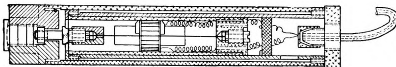
Фиг. 8. Струнный телетермометр проф. Н. Н. Давиденкова.
