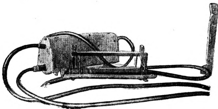
Фиг. 3. Телетензометр для измерения температурных деформаций. На переднем плане — справа — прибор без кожуха; слева — прибор в кожухе, готовый к установке.
