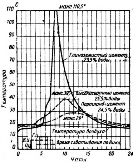
Фиг. 46. Кривые повышения температуры после затворения для различных цементов. (Из работ механической лаборатории в Цюрихе.)
