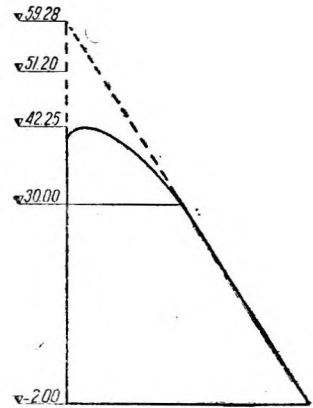
Фиг. 12: Заменяющий треугольный профиль при расчете по методу акад. Б. Г. Галеркина.
