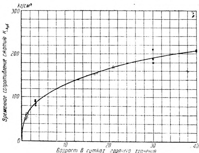
Фиг. 21. Результаты испытаний контрольных кубиков бетона.
