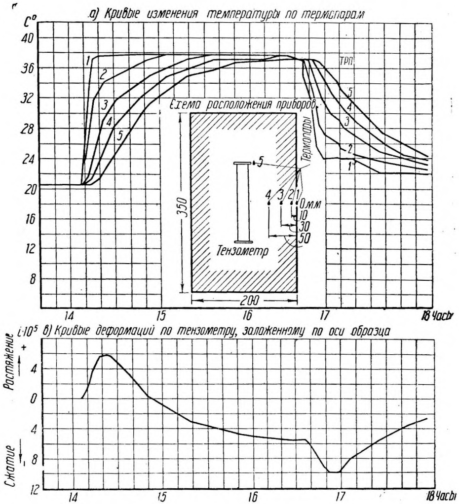
Фиг. 1. График изменения температур и деформаций в призме 20 x 20 X 35 см при погружении в горячую и холодную ванну.
