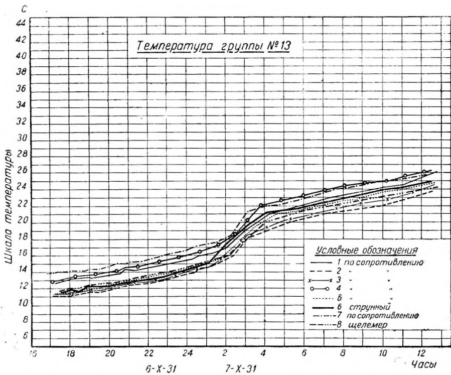
Фиг. 50. График изменения температуры после укладки бетона в группе № 13.
