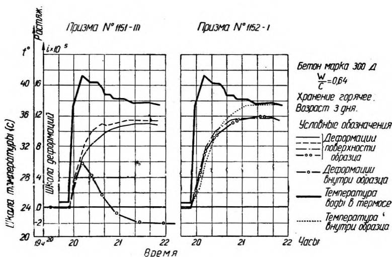
Фиг. 6. Графики деформаций бетонной призмы при изменении температуры.
