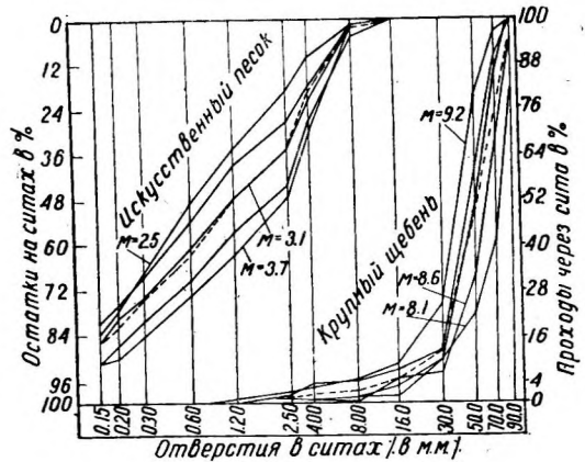
Фиг. 3. Кривые просеивания искусственного песка и крупного щебня.
