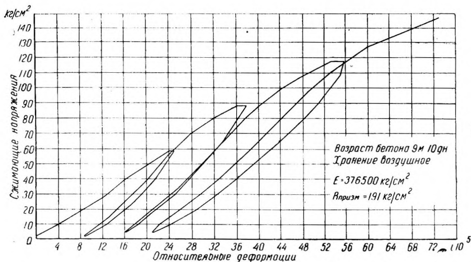
Фиг. 24. Кривые деформаций призмы (9,2 x 10,2 x 30 см) из бетона, выбуренного из плотины.
