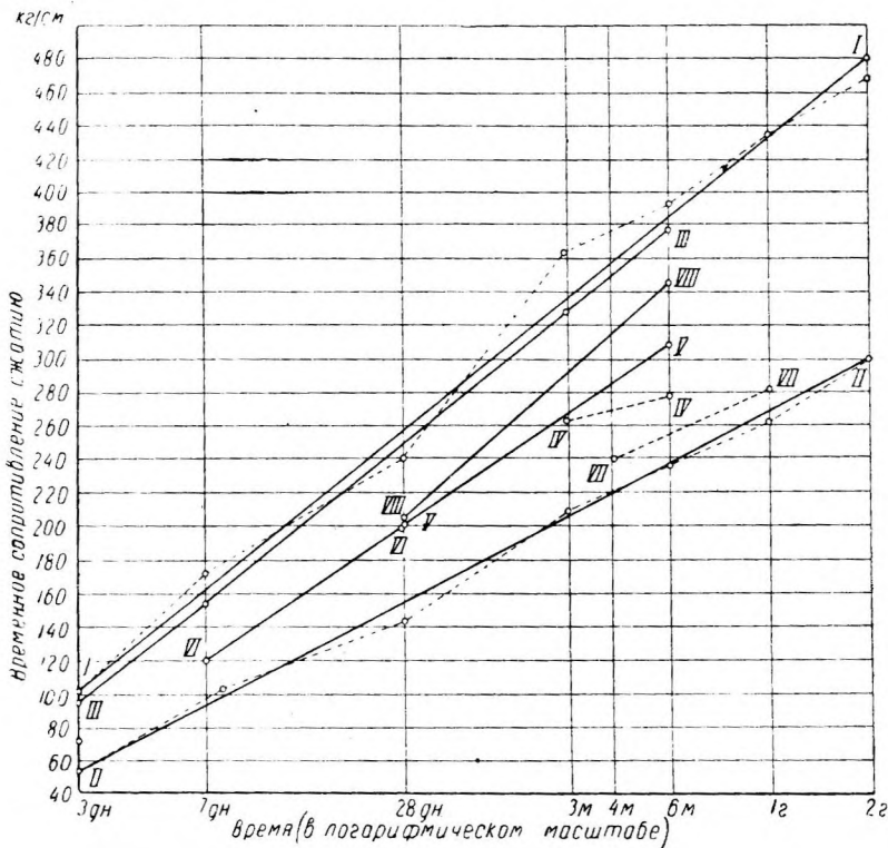
Фиг. 4. Рост кубиковой прочности бетона со временем.
