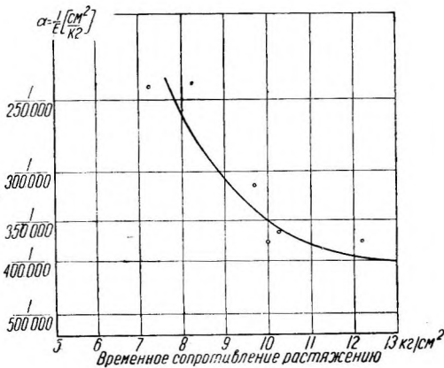
Фиг. 25. Зависимость модуля упругости бетона при растяжении от временного сопротивления.
