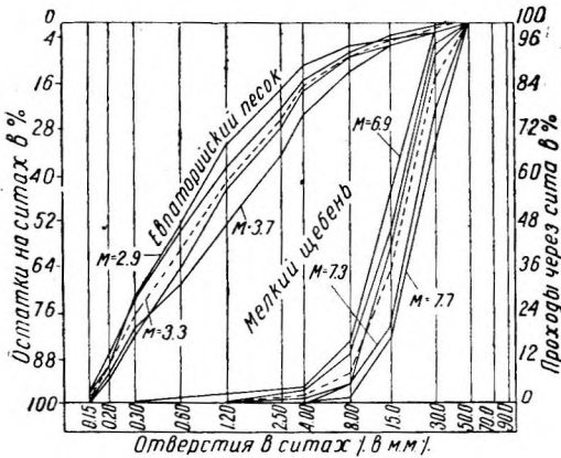
Фиг. 2. Кривые просеивания евапаторийского песка и мелкого щебня.
