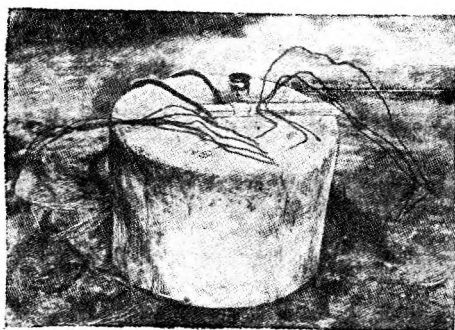
Фиг. 4. Установка термопар на поверхности образца для проверки изоляции.
