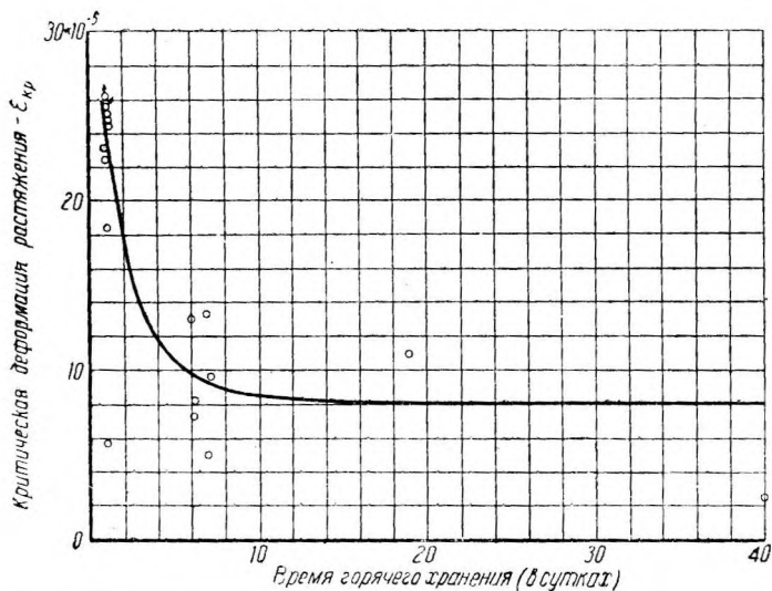
Фиг. 22. Зависимость критических деформаций при растяжении бетона от возраста.
