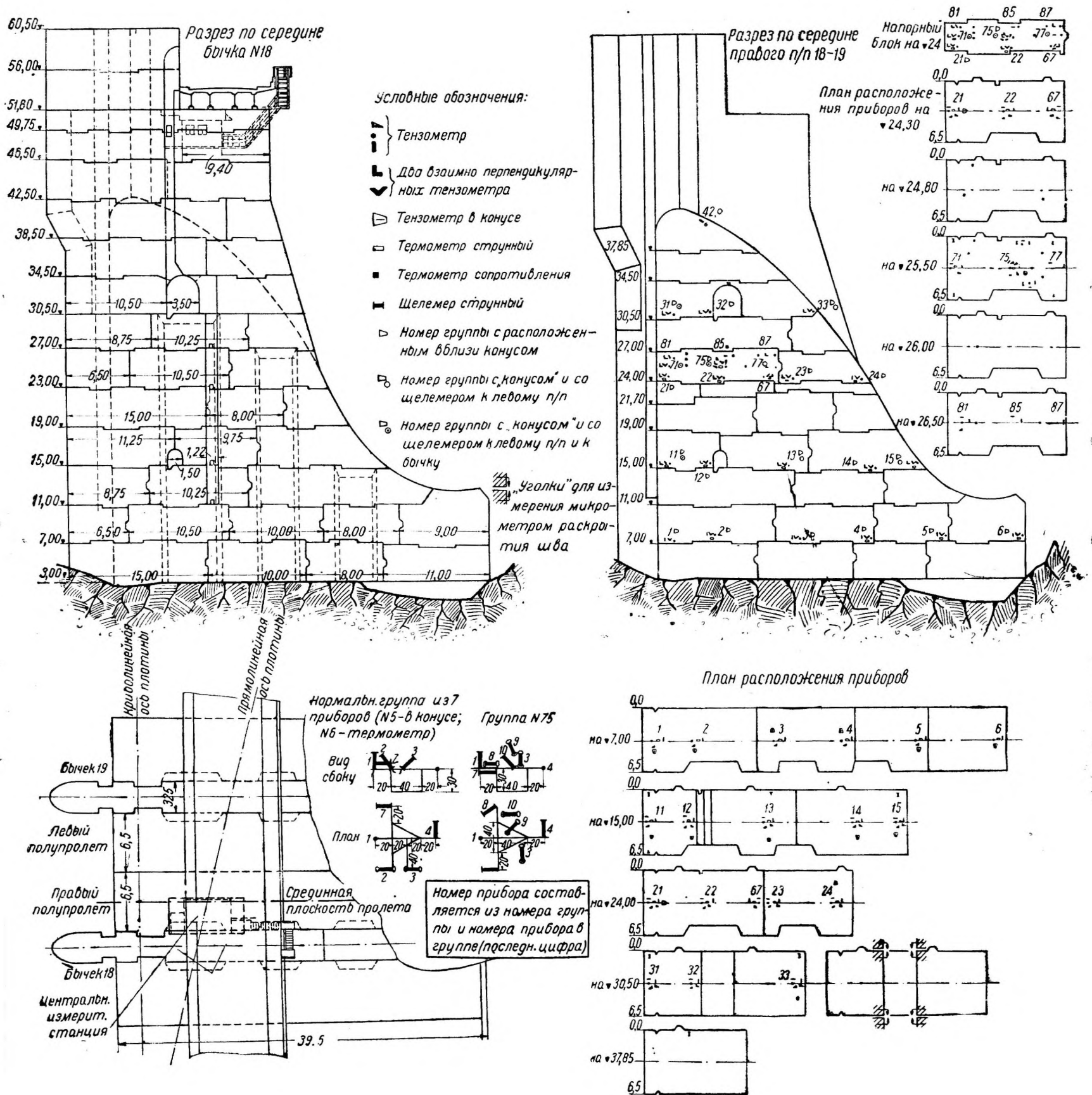
Фиг. 1. Схема размещения приборов по профилю плотины.
