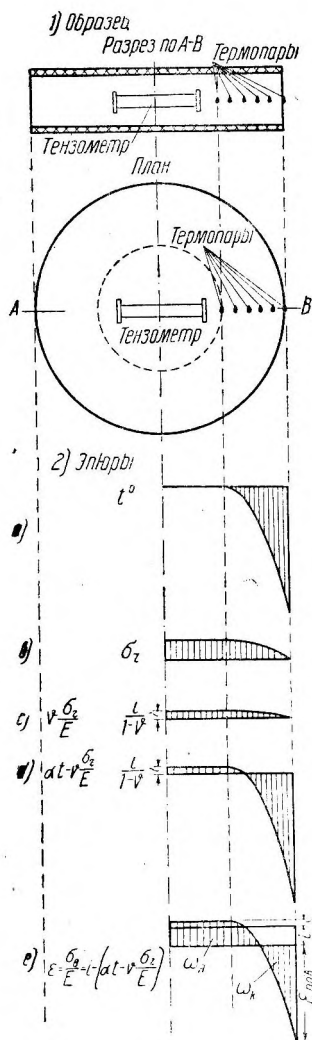
Фиг. 8. Схема измерения деформаций и температур.
