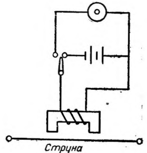
Фиг. 1. Принципиальная схема способа Шефера.
