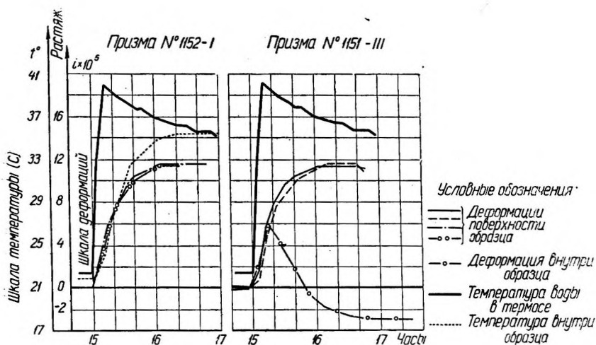
Фиг. 7. Графики деформаций бетонной призмы при изменении температуры. Бетон марок 285Д и 300Д. Хранение влажное при +40° и нормальное; \frac{W}{C} = 0,62 - 0,64 .
