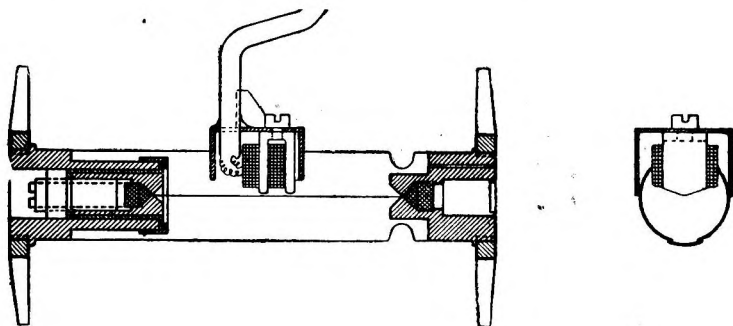
Фиг. 5. Струнный телетензомер проф. Н. Н. Давиденкова (модель 1930 г.).
