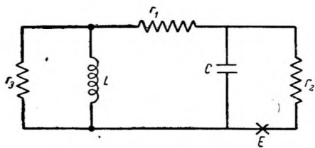
Фиг. 5. Эквивалентная схема генератора Лазарева.
