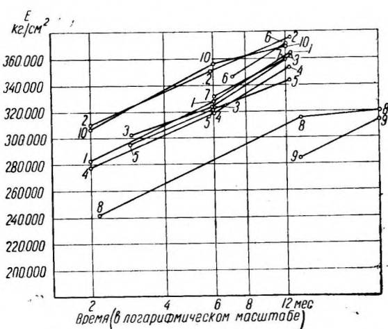
Фиг. 20. Рост модуля упругости при сжатии со временем для бетона марки 300Д. Состав по весу 1 : 2,58 : 4,23; \frac{W}{C} = 0,55-0,58 . Хранение во влажных опилках.
