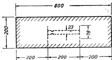
Фиг. 1. Призма с заложным внутри ее телетензометром.
