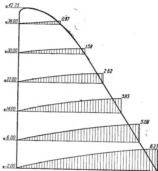
Фиг. 7. Эпюры скальвающих напряжений \tau по горизонтальным сечениям для второй схемы загрузки (собственный вес и давление воды при отметке горизонта 51, 20). Напряжения в кг/см^2 .
