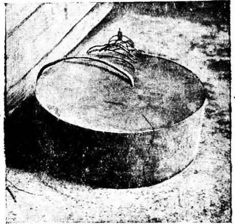
Фиг. 12. Внешний вид образца с трещиной, составляющей угол около 60° с осью прибора.
