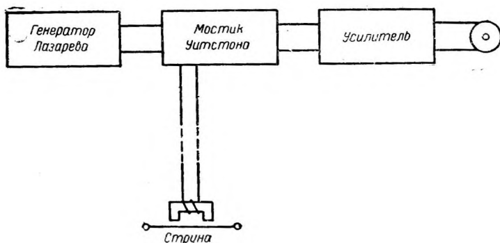
Фиг. 10. Схема установки 1931 г.
