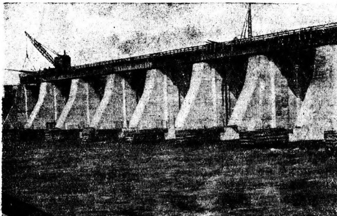
Фиг. 17. Ряжи под эстакаду на носгах бычков (1930 г.).
