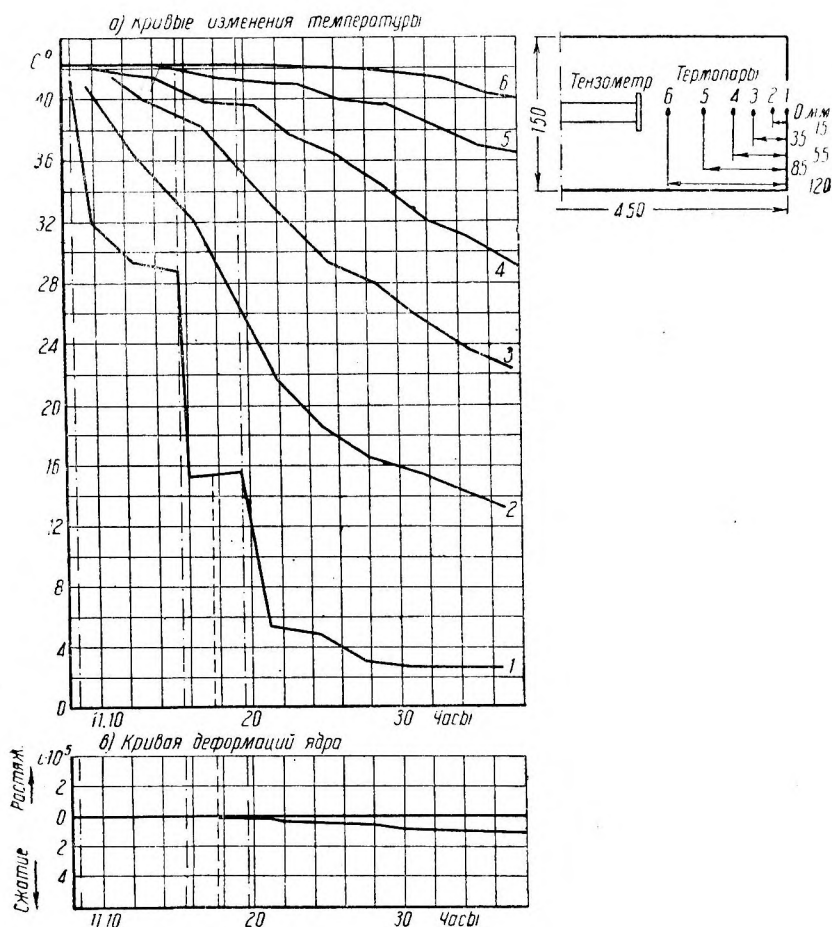
Фиг. 13. Влияние поверхностной трещины на деформации ядра.
