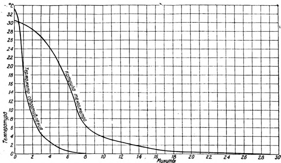
Фиг. 18. Сравнительная характеристика тепловой инерции термометра сопротивления и катушки телетензомера.
