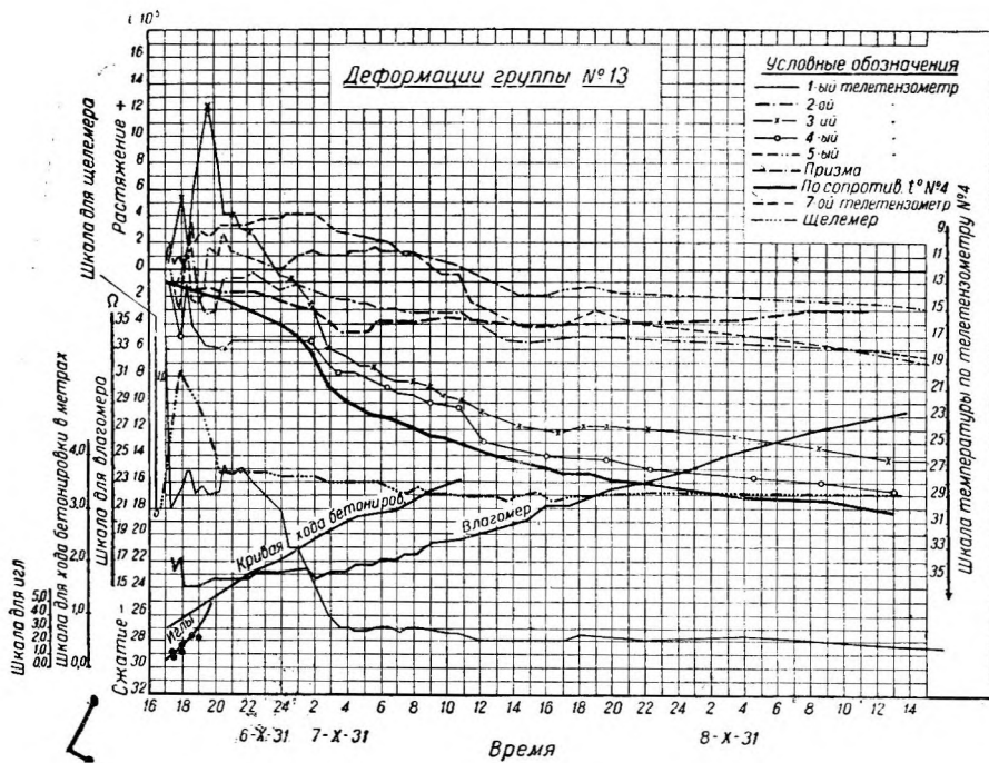
Фиг. 49. Полевой график наблюдений по приборам.
