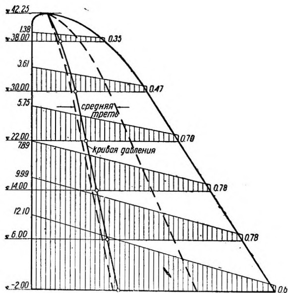
Фиг. 2. Кривая давления и эпюры нормальных напряжений \sigma_y для первой схемы загрузки (только собственный вес). Напряжения в \text{кг}/\text{см}^2 .
