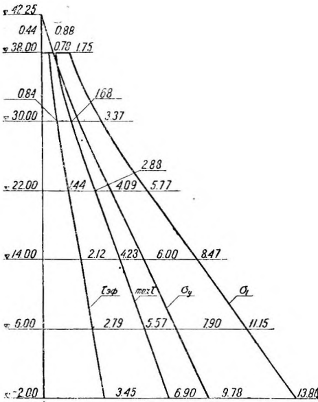
Фиг. 11. Эпюры наибольших напряжений (в \text{кг/см}^2 ) по низовой грани для второй расчетной схемы загрузки.
