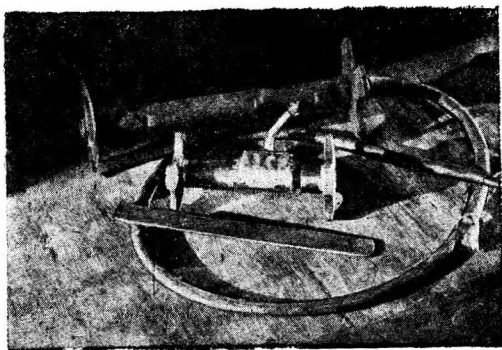
Фиг. 11. Внешний вид телетензографов (модели 1930 и 1931 гг.)
