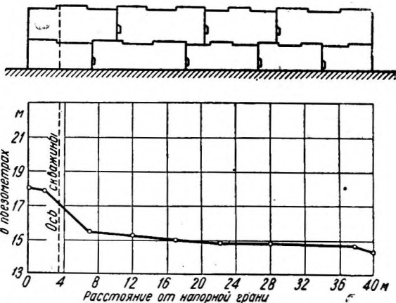
фиг. 6. Эпюра распределения гидростатического давления под основанием плотины (по промеру от 7/IX 1931 г.)
