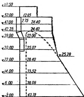
Фиг. 13. Расчетный профиль бычка плотины (размеры в м)
