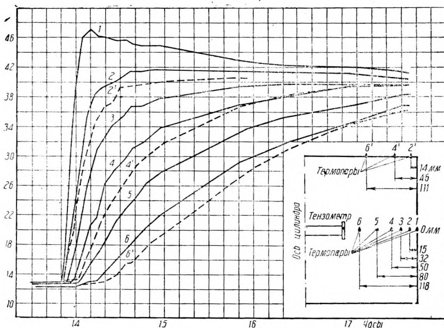
Фиг. 3. Графин изменения температуры в срединном и торцевом сечении образца с тепловой изоляцией.
