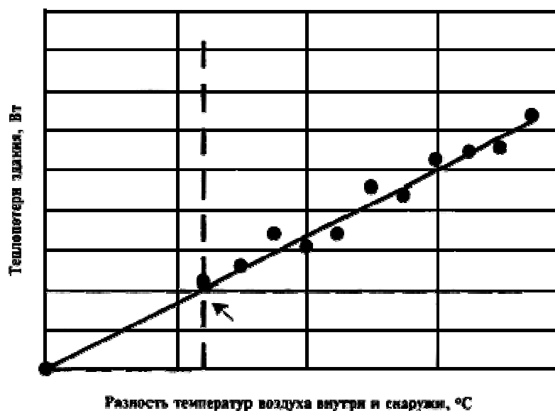
Рисунок 1 - Схема функциональной зависимости теплотеря здания от разности температур воздуха внутри и снаружи
