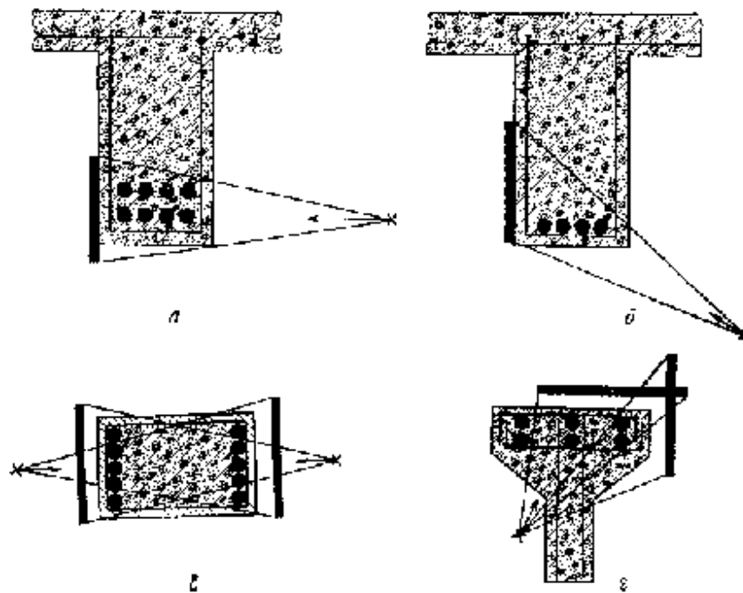
а - балка ребристого перекрытия при двухрядном расположении арматуры; б - то же, при однорядном расположении; в - колонна; г - сборная балка
