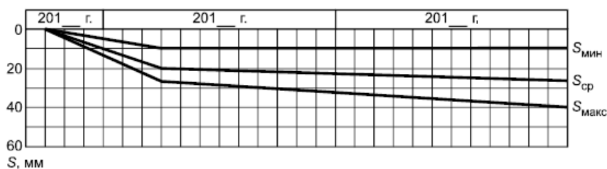
Рисунок Б.4 - График развития перемещений
