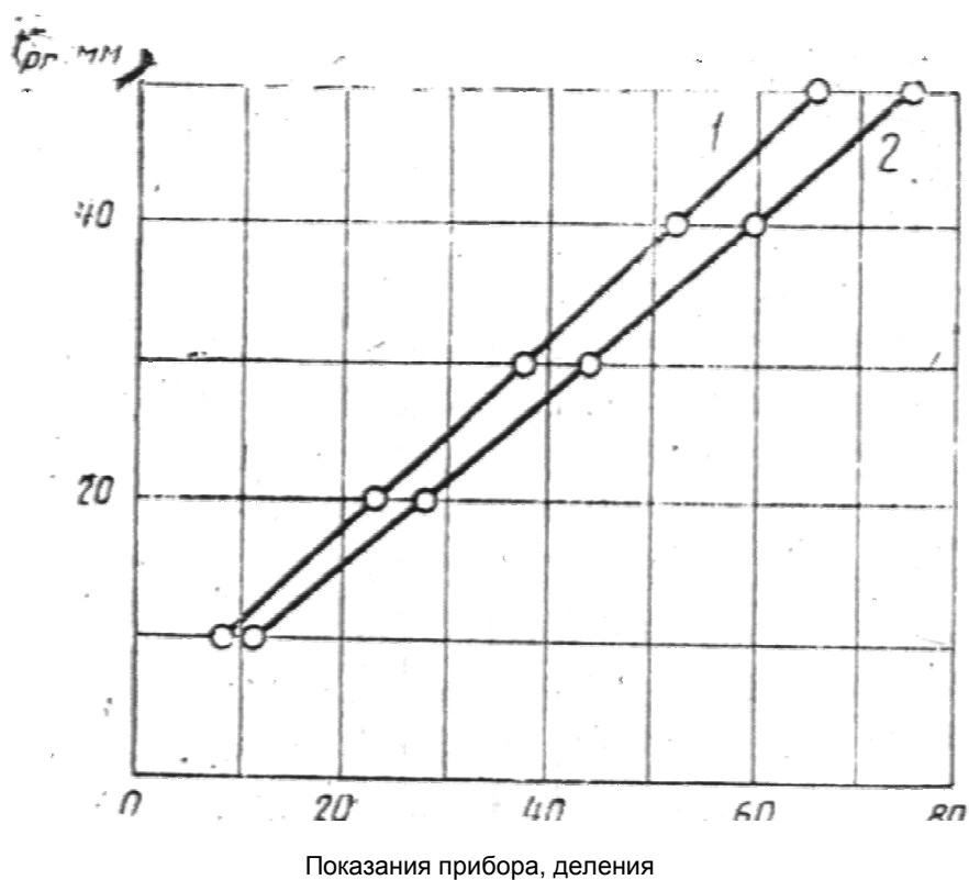
Чертеж В.1 - Градуировочные зависимости для продольных стержней диаметром 16 мм
