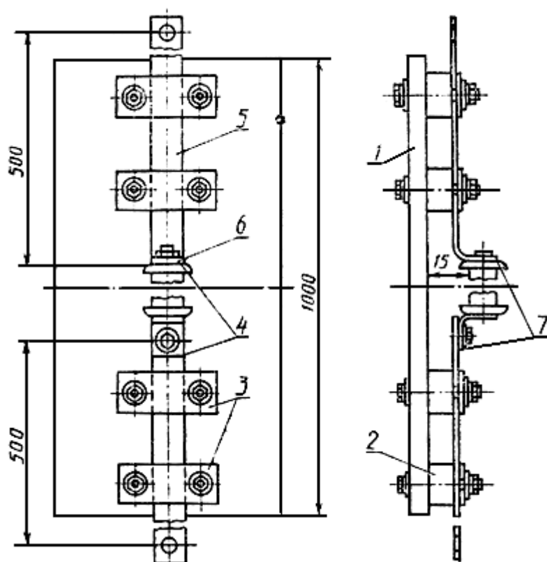
1 - изоляционное основание; 2 - изолятор; 3 - изолированные скобы; 4 - луженая контактная поверхность; 5 - матовая поверхность черного цвета; 6 - место установки термопар; 7 - точки измерения напряжения.
