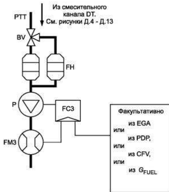
Рисунок Д.14 - Система отбора проб вредных частиц
